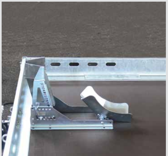
Radstopper für Motorräder
