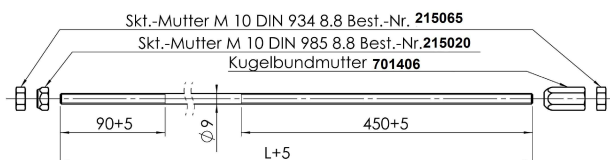
Bremsgestänge Ø 9
