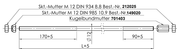
Bremsgestänge Ø 12
